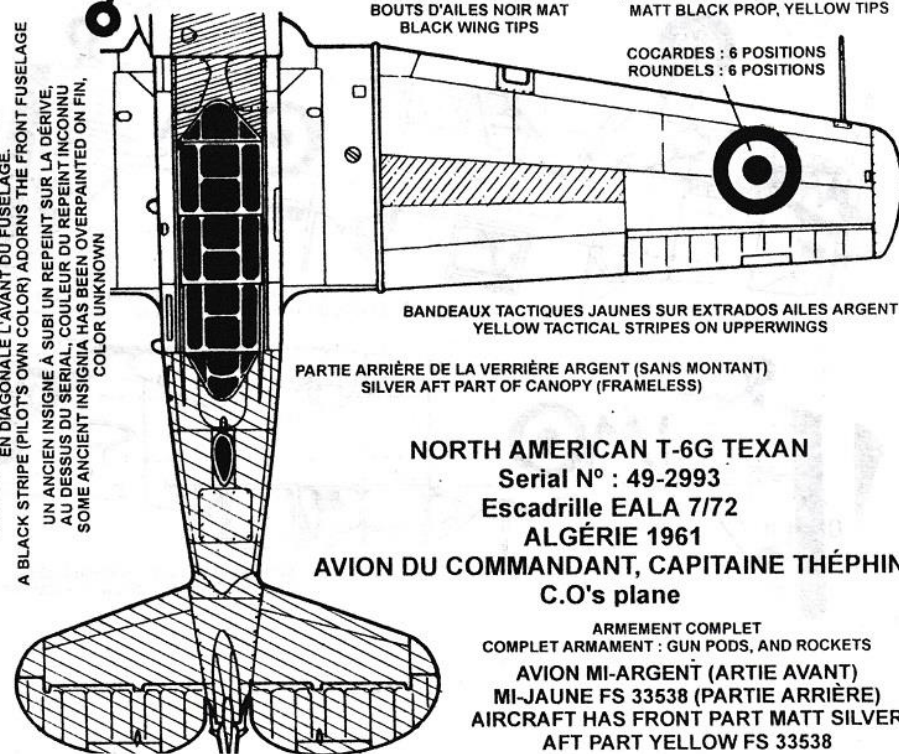
HÉLICE NOIR MAT, POINTES JAUNES MATT BLACK PROP, YELLOW TIPS
