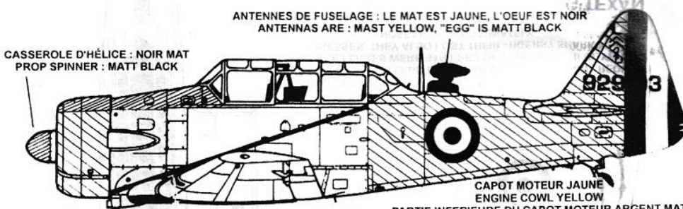
CAPOT MOTEUR JAUNE ENGINE COWL YELLOW PARTIE INFÉRIEURE DU CAPOT MOTEUR ARGENT MAT ENGINE COWL UNDER PANNEL IS SILVER
