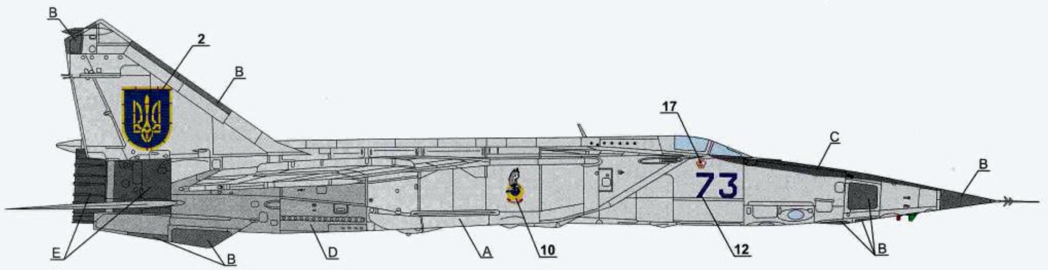
4. MiG-25RBТ Blue 73, 48th SGRAR Ukrainian Air Force, ZARP, Zaporozhye, early 2000s 4. МiГ-25РБТ б/н 73, 48 ОГРАП ПС України, ЗАРЗ, Запоріжжя, початок 2000-х
