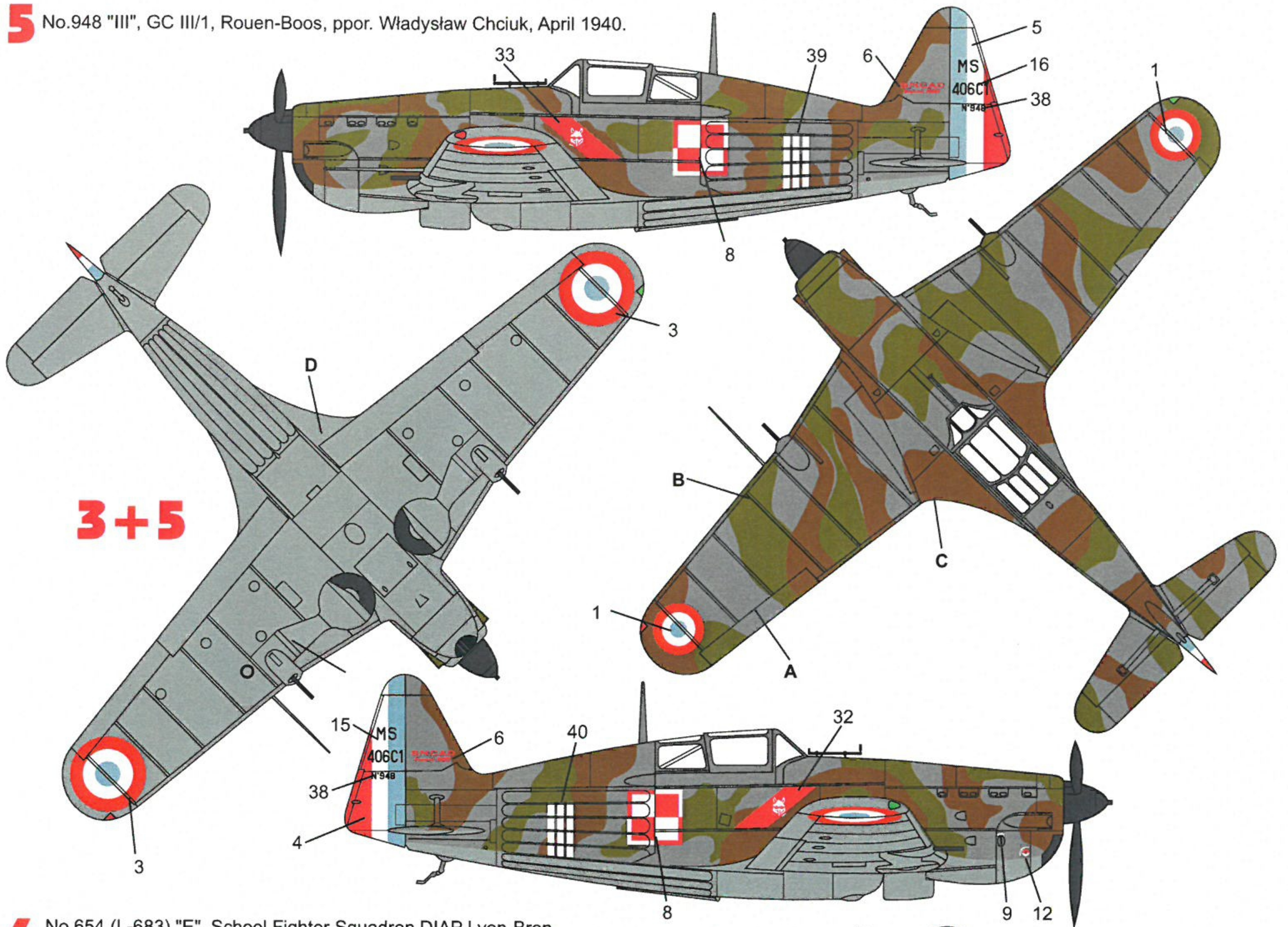
6 No.654 (L-683) "E", School Fighter Squadron DIAP Lyon-Bron, ppor. Wacław Król, ppor. Stanisław Chałupa, sierż. Leopold Flanek, spring 1940.
