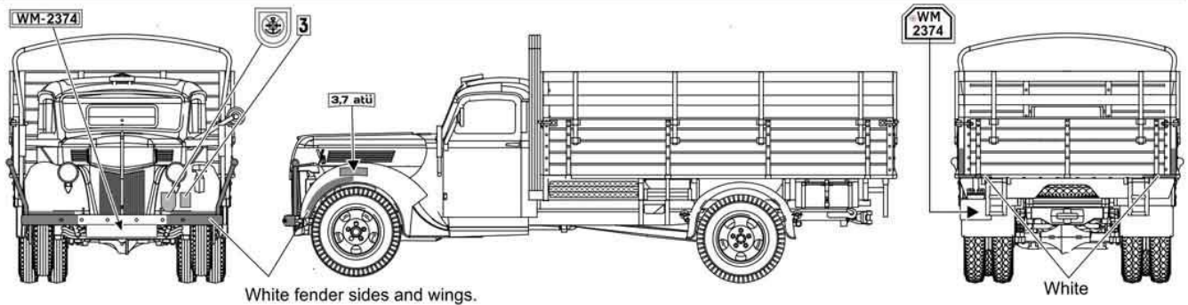
V3000S 3t German Cargo truck. Unidentified Kriegsmarine unit. Panzer Grey (RAL 7021). 1942. V3000S немецкая трёхтонка. Неустановленное подразделение Кригсмарине. Panzer Grey (RAL 7021). 1942.
