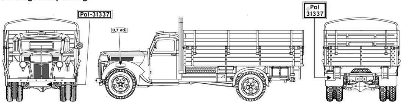
V3000S 3t German Cargo truck. German Ordnungspolizei. Central Europe. Overall Green (RAL 6009). 1943. V3000S немецкая трёхтонка. Полиция Германии. Центральная Европа. Глянцевый зелёный. (RAL 6009). 1943.
