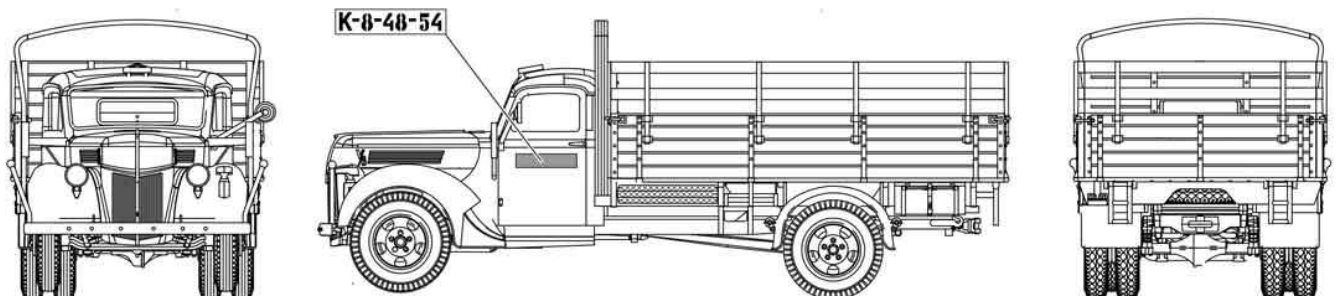
V3000S 3t German Cargo truck. Red Army war Trophy. Soviet Khaki (4B0). 1944. V3000S немецкая трёхтонка. трофей Красной Армии. Советский хаки (4B0). 1944.
