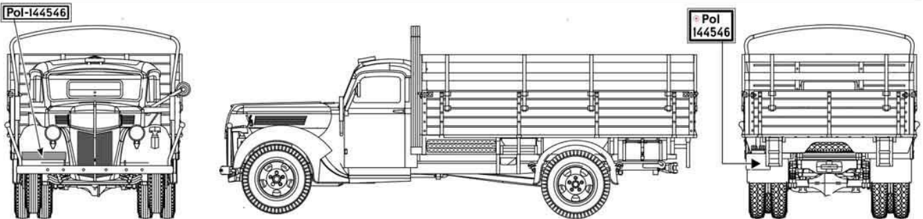
V3000S 3t German Cargo truck. German Ordnungspolizei. Central Europe. Overall Green (RAL 6009). 1943. V3000S немецкая трёхтонка. Полиция Германии. Центральная Европа. Глянцевый зелёный. (RAL 6009). 1943.
