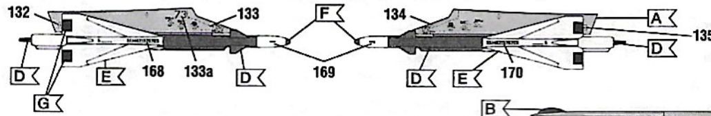
right pylon inside / rechter Pylon Außenseite
