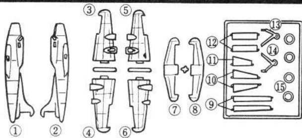
胴体部品番号図 Parts
