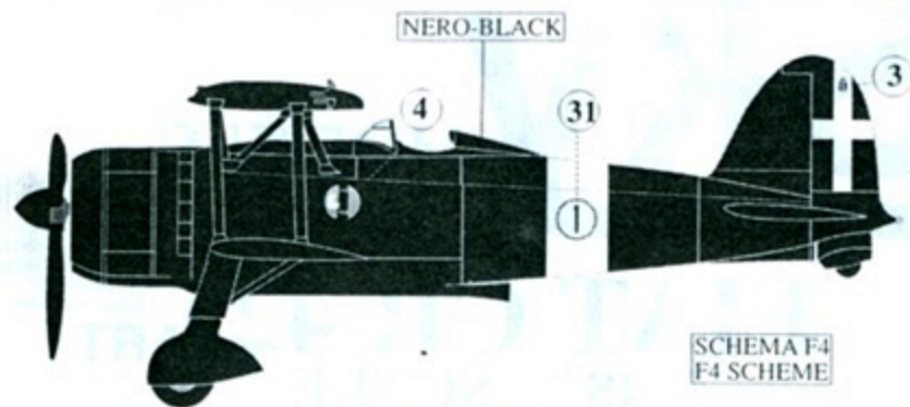
Fiat CR 42 serie XIII, Nucleo Aut. Caccia Notturna, Gela, Autunno 1942
