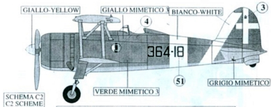
Fiat CR 42, 364 o Sq.150 o Gr.53 o St.C.T. Valona,Dicembre 1940
