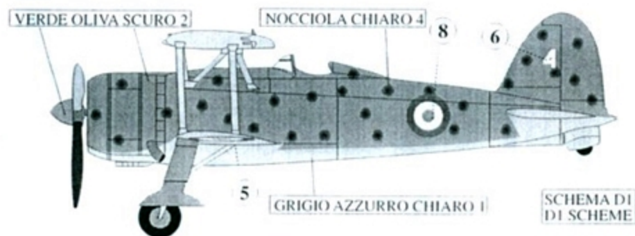
Fiat CR 42, Sezione Autonoma Collegamenti, Roma-centocelle, Inverno 1945-1946
