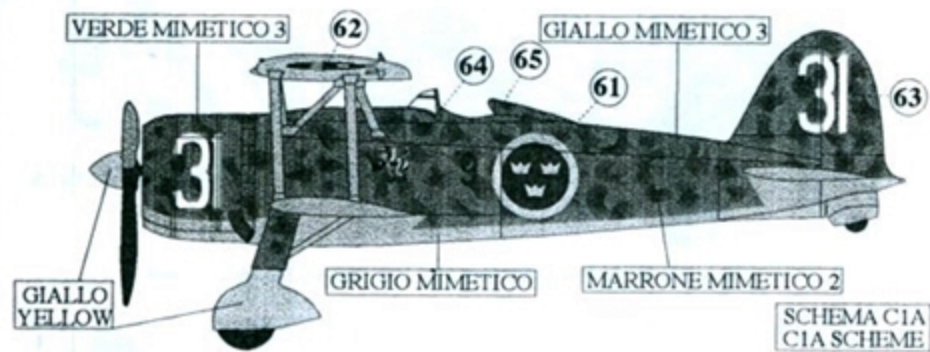
Fiat J.11(CR 42) n. 2541, Divisioni 3, Kungliga Gota Flygflottilj F9, Svenska Flygvpnnet, Sac, Marzo 1942
