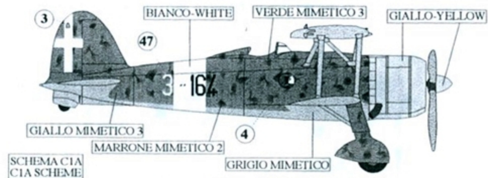
Fiat CR 42,164 a Sq.161 o Gr. Aut.C.T.Rodi, 1941
