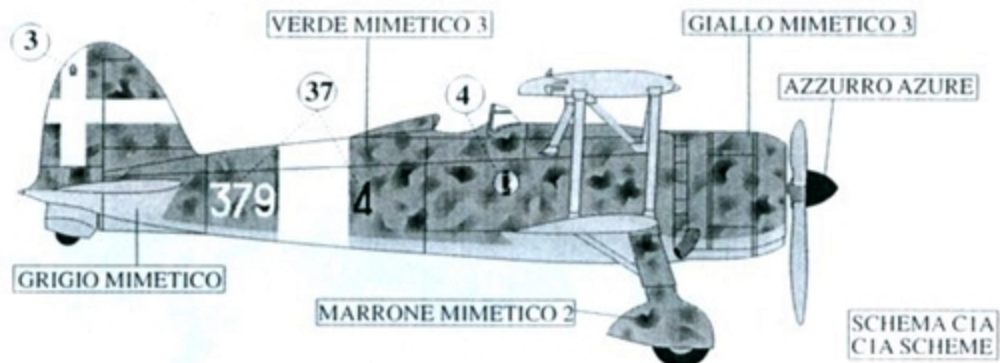
Fiat CR 42 ,379 o Sq. ,156 o Gr.Aut. C.T., Comiso ,Febbraio 1941
