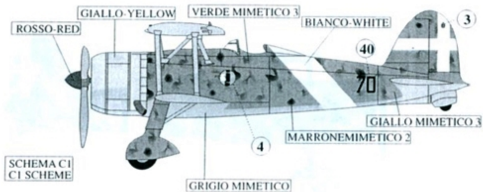
Fiat CR 42, - 23° Gr.Aut. C.T. Maggiore Tito FALCONI, Trapani - Milo, Luglio 1941
