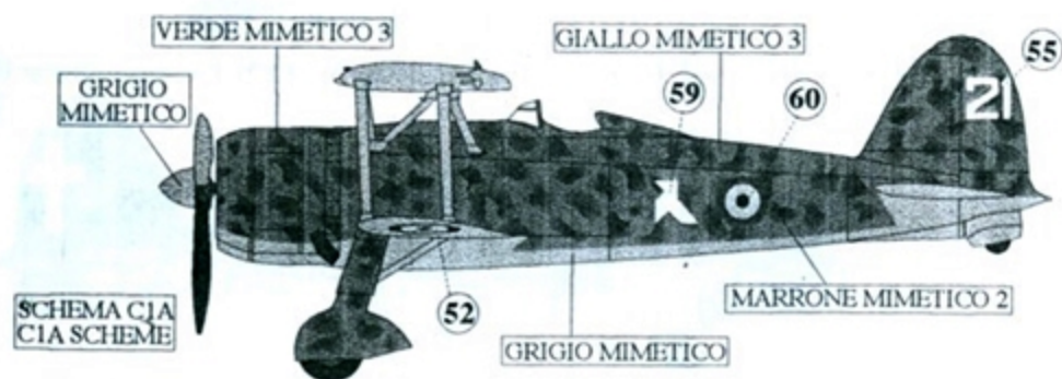
Fiat CR 42, matricola R.21, 4 a Escadrille, 11e Groupe, 2e Regiment, Aeronautique Militaire Belge, Brustem , Maggio 1940
