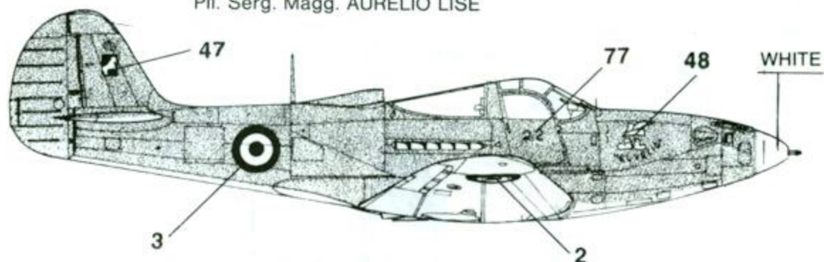
BELL P 39L AIRACOBRA 9° Gr. 4° St. C.T. (Leverano 1944) Pil. Serg. Magg. AURELIO LISE
