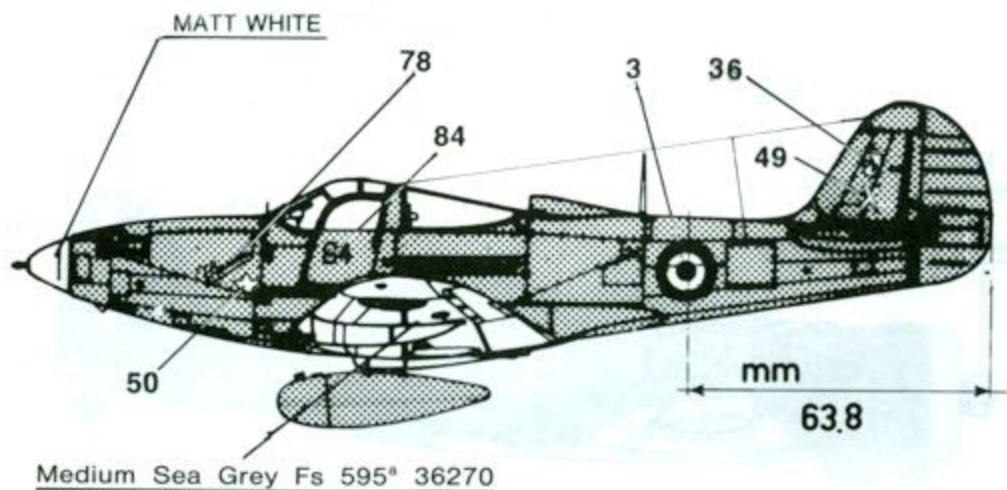
BELL P 39Q AIRACOBRA 10° Gr. 4° St. C.T. (Termoli 1945)
