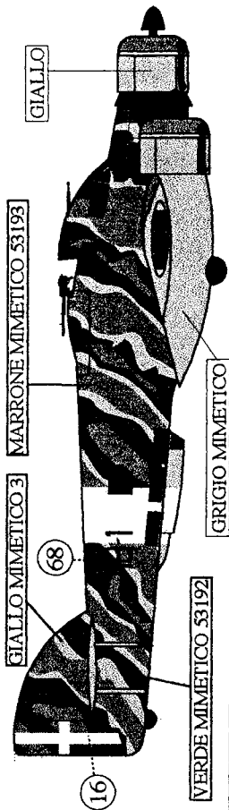
SAVOIA MARCHETTI SM 79 - 18°Sq. 27° Gr. 8° St. Primavera 1941
