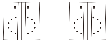
水听孔定位 (1:1)
