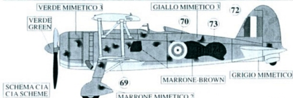
Fiat CR 42, BT 474 (ex MM.5701 della 95 o Sq.)R.A.F.Martlesham Heat,UK, novembre 1940
