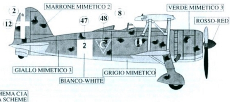
Fiat CR 42, 377 a Sq. Aut. Intercettori, Palermo, Luglio 1942
