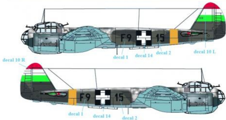
F.9+15: Junkers Ju-88 D-1, 1/1 Távolfelderítő század (Long Range Reconnaissance Squadron) Harkov, 1943. Plane of Főhadnagy Visnyei
